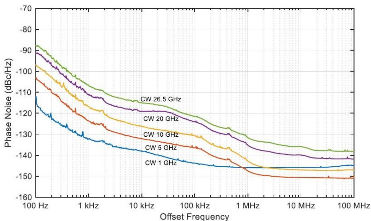
配置选件 012 的相位噪声，端口 1&3，源 2 输出 1—典型值
